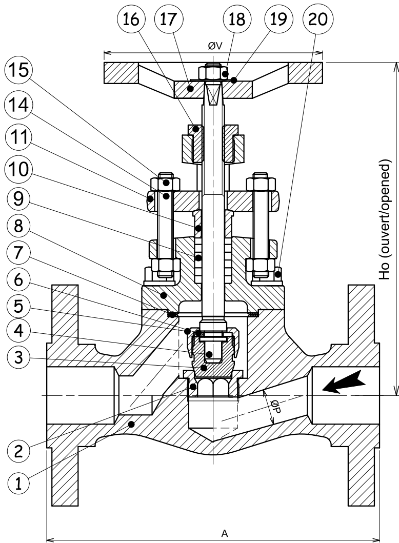
CHAPEAU BOULONNÉ / BOLTED BONNET SIÈGE VISSÉ / RENEWABLE SEAT
