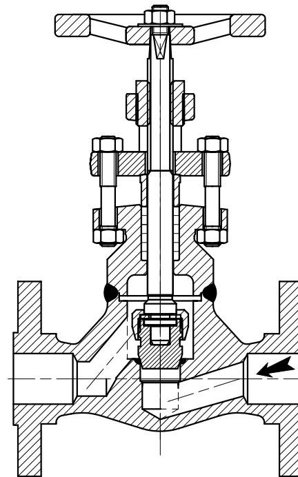
CHAPEAU SOUDÉ / WELDED BONNET SIÈGE INTÉGRAL / INTEGRAL SEAT
